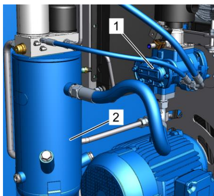
Рис. 17: Ступень компрессора
