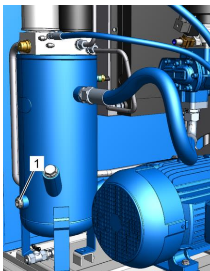
Рис. 32: Проверка уровня охлаждающей жидкости через смотровое отверстие
