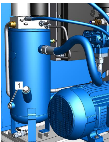
Рис. 30: Смотровое отверстие
