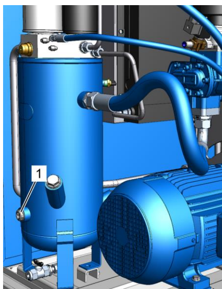
Рис. 39: Смотровое отверстие
