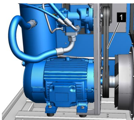
Рис. 15: Приводной агрегат
