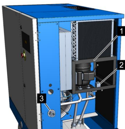
Рис. 23: Рефрижераторный осушитель
